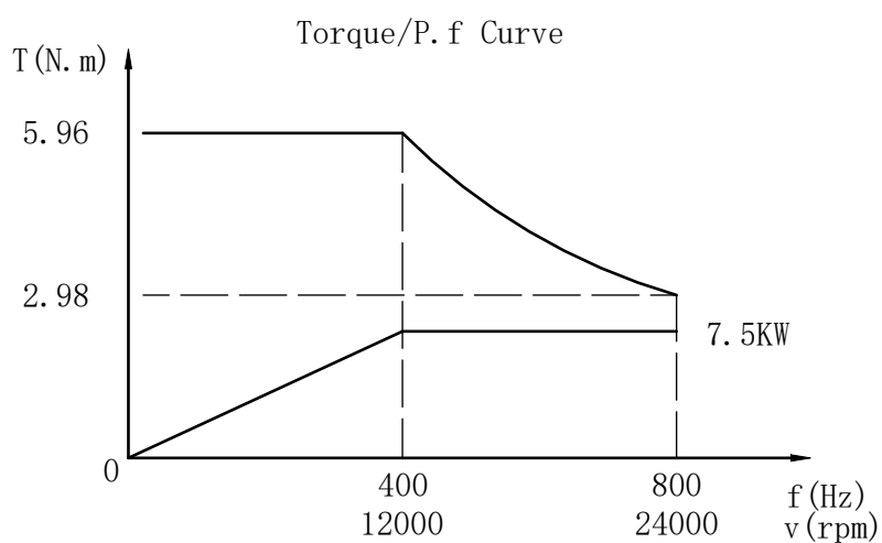
扭矩/功率曲线
