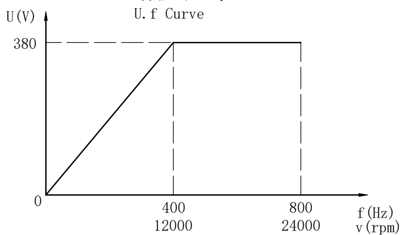
频压曲线
